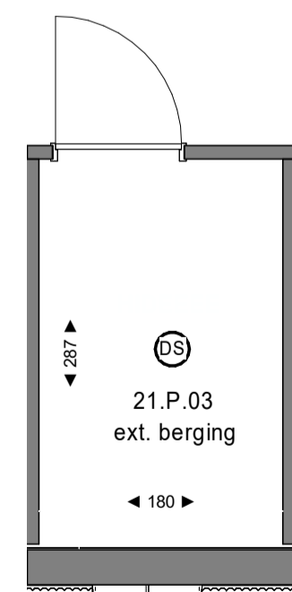
plattgrond berging 1 : 50 4e verdieping
