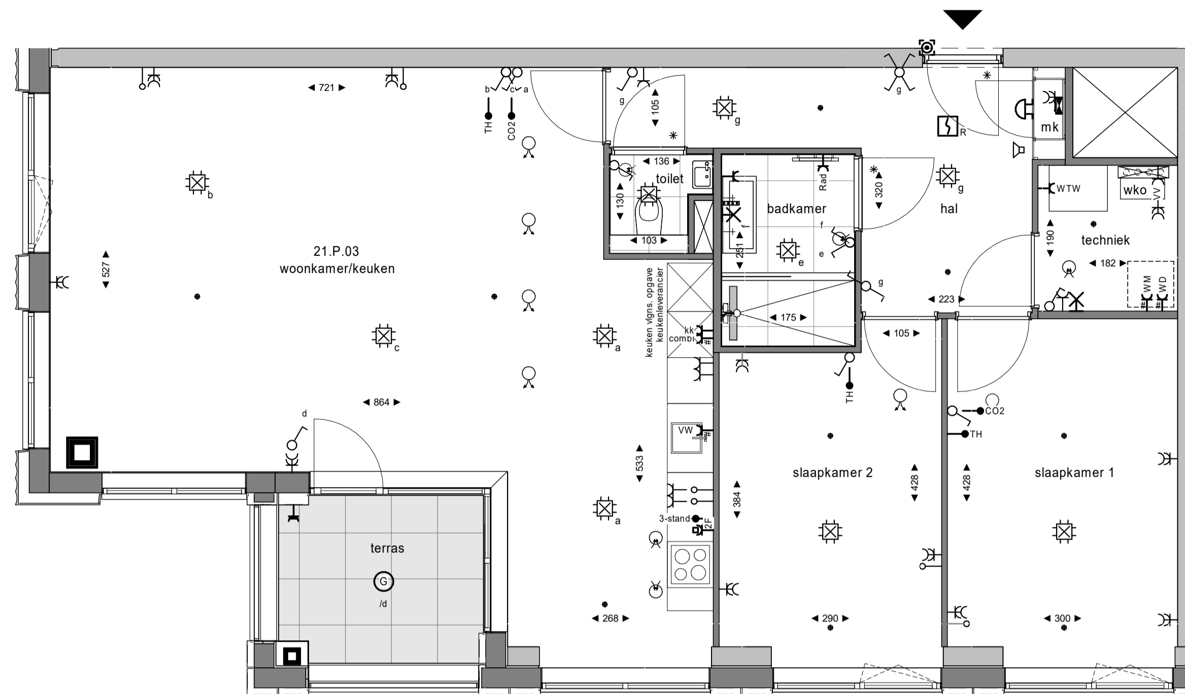
plattgrond 1 : 50 21e verdieping
